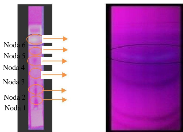
Gambar I. Hasil KLT dan KLT preparatif dengan eluen n-heksan:etil asetat: etanol (30:2:1)
