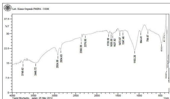
Gambar IV. Spektogram FTIR isolat alkaloid daun tempuyung
