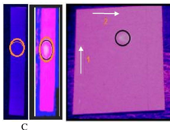
Gambar II. (A), (B) Hasil KLT dengan berbagai campuran eluen (C) KLT dua dimensi pada lampu UV \lambda_{365 \text{ nm}}
