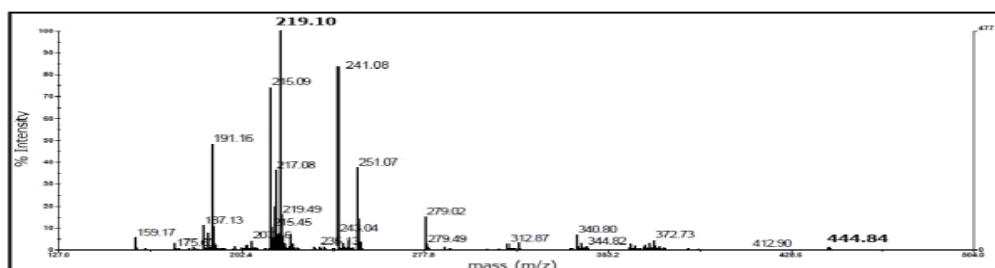
Gambar V. Spektrogram LC-MS isolat alkaloid daun tempuyung
